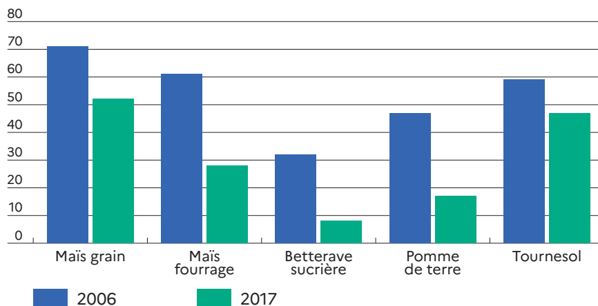
FIGURE 14 - PART DES SOLS NUS EN HIVER POUR PLUSIEURS CULTURES DE PRINTEMPS, DANS LES ZONES VULNÉRABLES, COMPARAISON 2006 – 2017 (MTES, 2008 ET OIEau, 2020) 21
