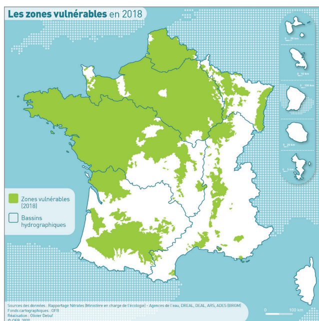
FIGURE 9 CARTE DES ZONES VULNÉRABLES EN VIGUEUR ZONAGE 2018 (OFB, 2020)
